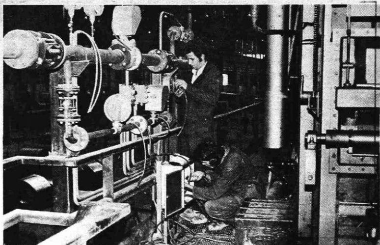
Montaža merilnih ur na liniji za silicijeva jekla v novi hladni valjarni.
