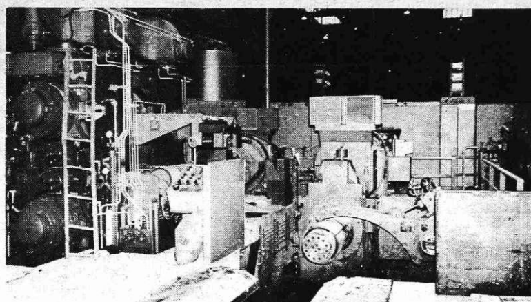
Nova hladna valjarna – mehansko testiranje dresirnega ogrodja.
