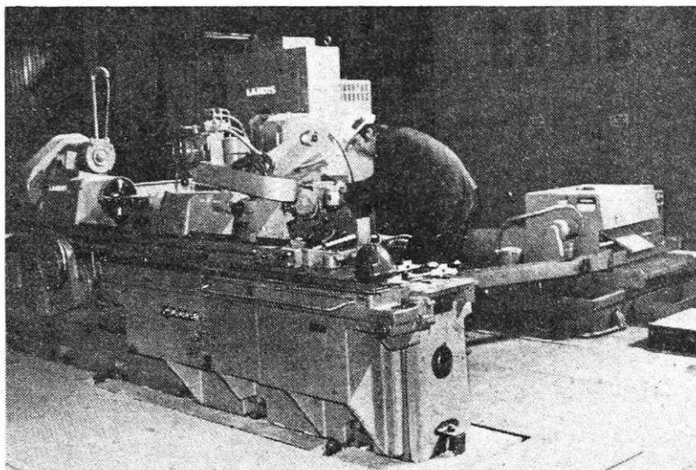
Montaža brusilnega stroja za sendzimir valje
