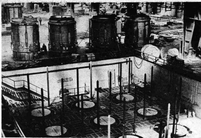
Zvonaste peči pripravljene za montažo
