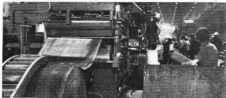
Testiranje Sendzimir valjavniškega ogrodja s pločevino
