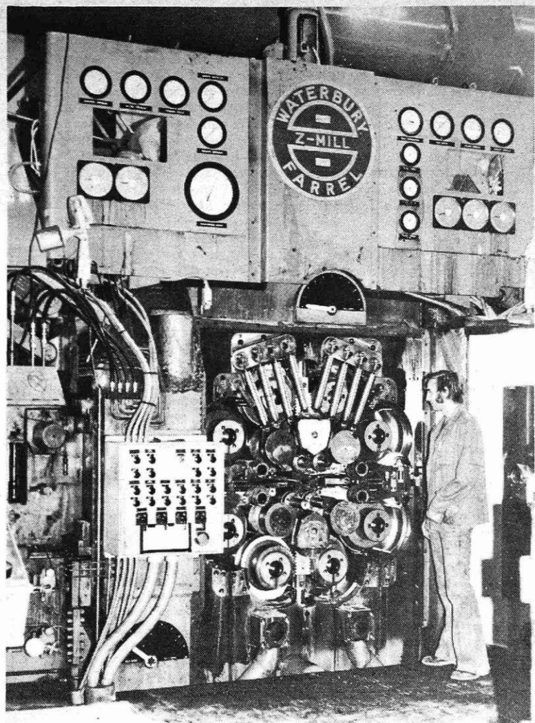
Notranjost sendzimirvaljavskega ogrođa z vloženimi valji, pripravljen za končno testiranje
