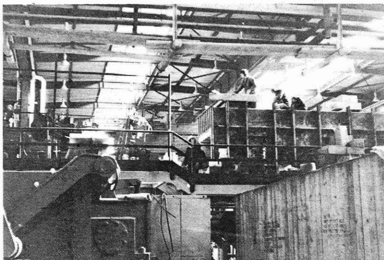
Obzidava peči na liniji za nerjavna jekla v novi hladni valjarni
