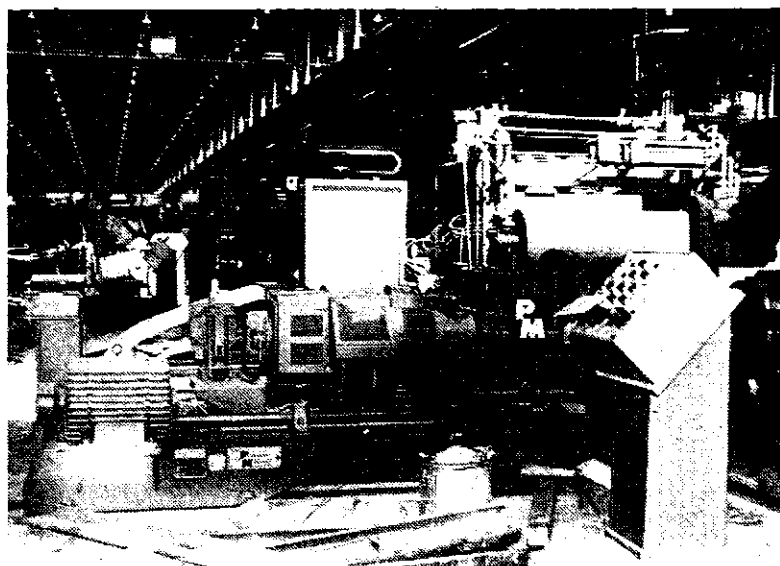
Testiranje linije za pripravo trakov
