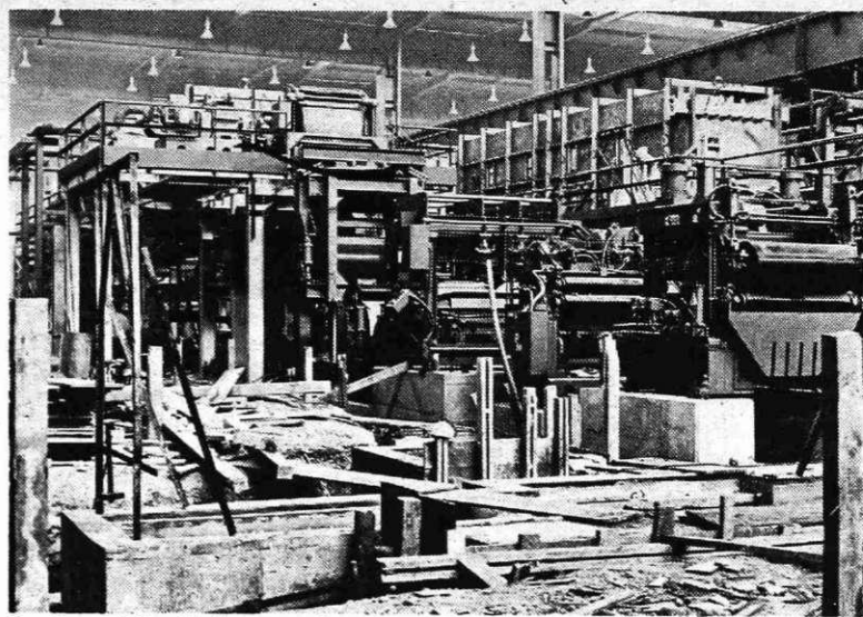
Žarilno lužilna linija za nerjavna in silicijeva jekla v novi hladni valjarni
