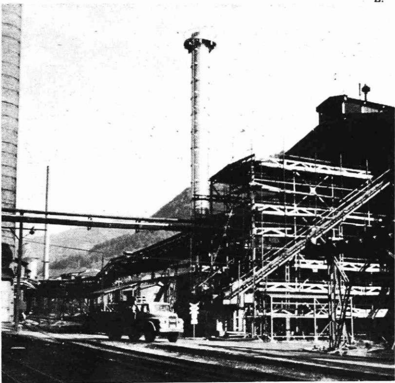
Izgradnja dimnika za vročevodni kotel za ogrevanje mesta Jesenice in Železarne
