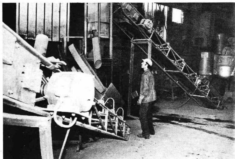
Polindustrijska linija za eksperimentalno proizvodnjo aglomeriranega varilnega praška
