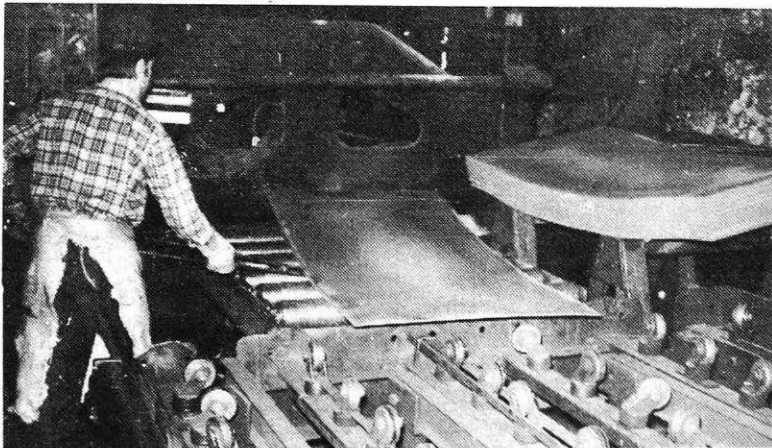
Sodelavec pri Demag ravnalnem stroju v valjarni debele pločevine.
