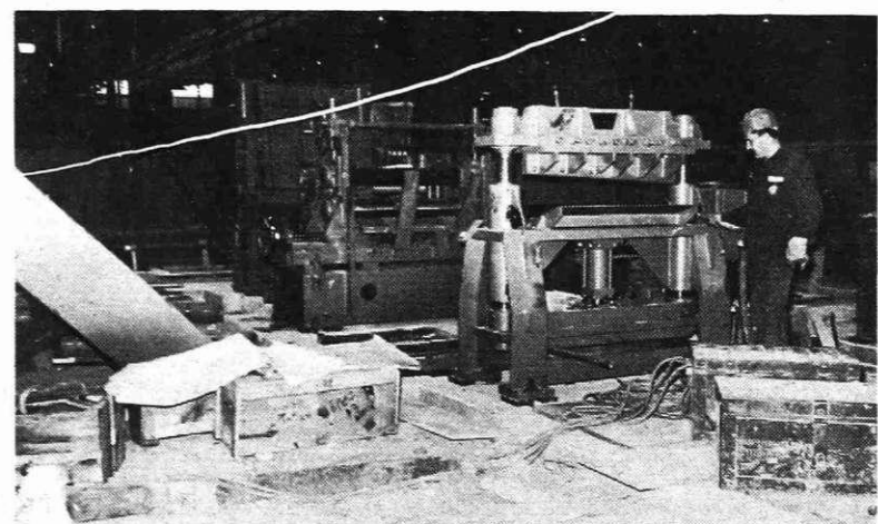
Vzdolžne škarje za razrez nerjavne pločevine v novi hladni valjarni
