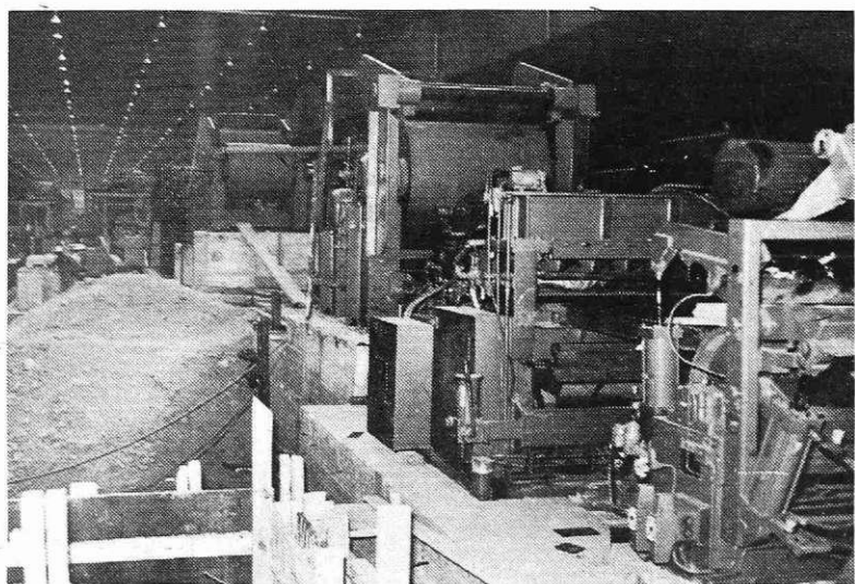
Izstopni del linije za pripravo trakov v novi hladni valjarni
