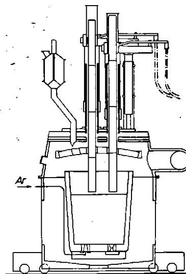
FINKL - MOOR vakumska naprava, najmlajša med tremi napravami, ki pridejo v poštev pri odločitvi v naši Železarni. Podroben opis in prednosti posamezne naprave lahko preberete v naši zadnji 14. številki Železarnja.
