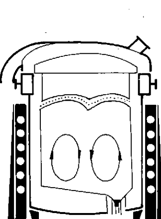
ASEA - SKF vakumska naprava, ki omogoča kakršenkoli metalurški postopek metalurške obdelave jekla izven tališniškega agregata.
