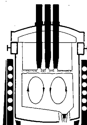
ASEA - SKF vakumska naprava, ki omogoča kakršenkoli metalurški postopek metalurške obdelave jekla izven tališniškega agregata.
