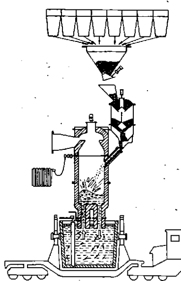
RH vakumska naprava, ena izmed treh tipov metalurških tehnoloških postopkov, med katerimi se bomo morali odločiti v Železarni, kot novem členu v naši kvalitetni usmeritvi
