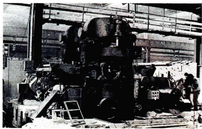
Montaža dresirnega ogrodja v novi hladni valjarni
