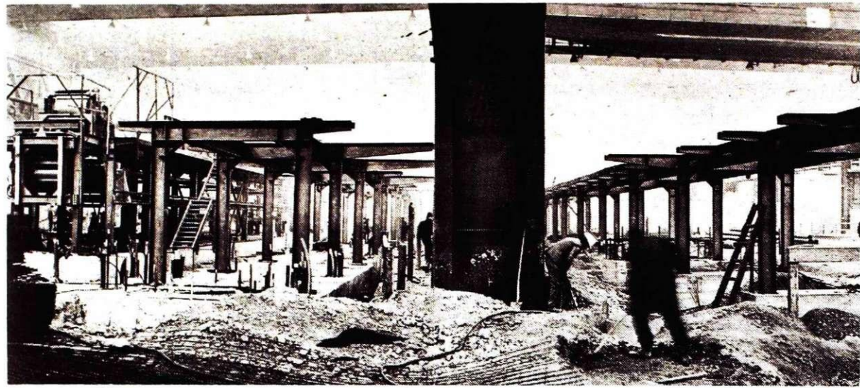
Montaža žarilno lužilne linije za mehka, nerjaveča in silicijeva jekla
