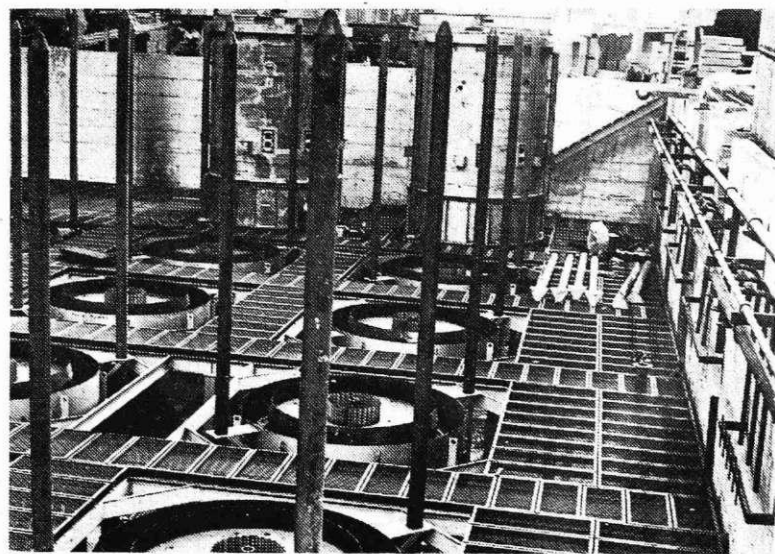
Zvonaste peči v novi hladni valjarni
