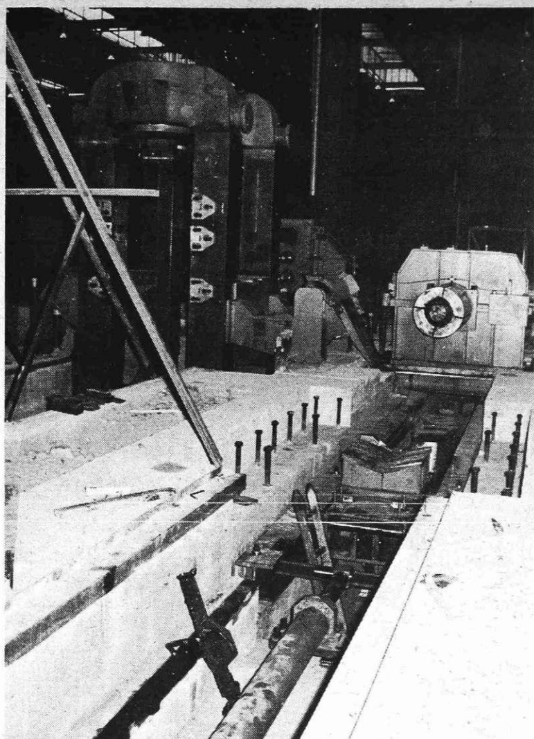
Montaža drsirnega ogrodka v novi hladni valjarni
