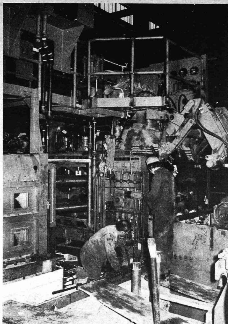
Montaža sendzimir ogrodja v novi hladni valjarni
