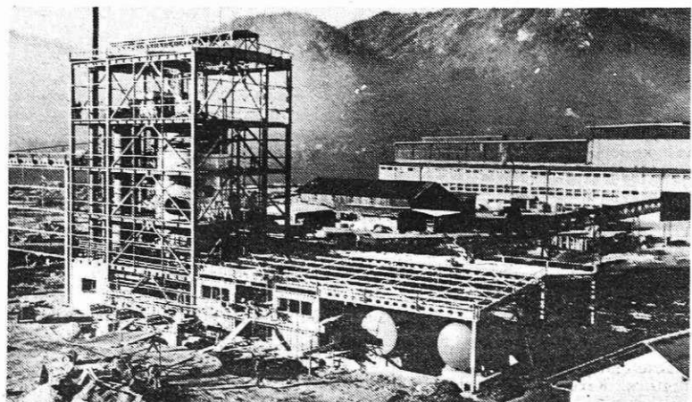
Nova hladna valjarna — gradnja objekta regeneracije
