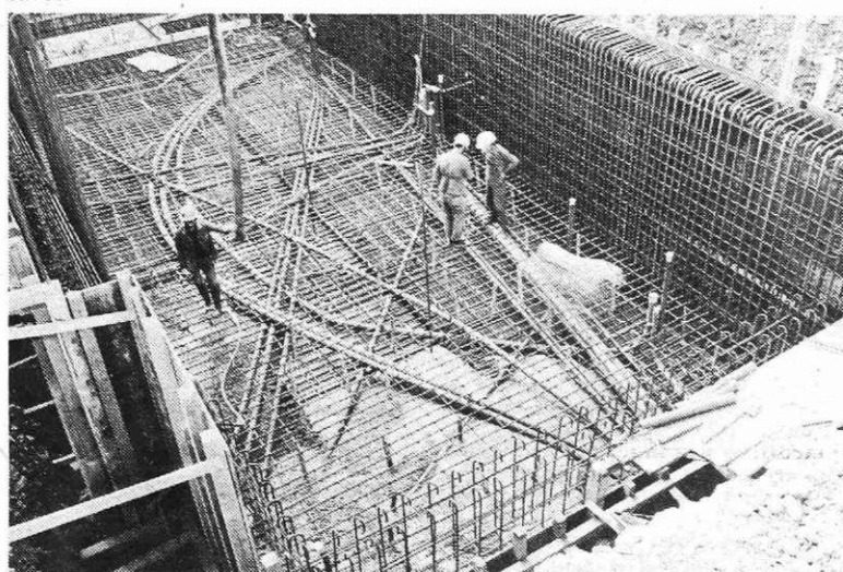
Polaganje cevi za GPL – BRUSILNA LINIJA
