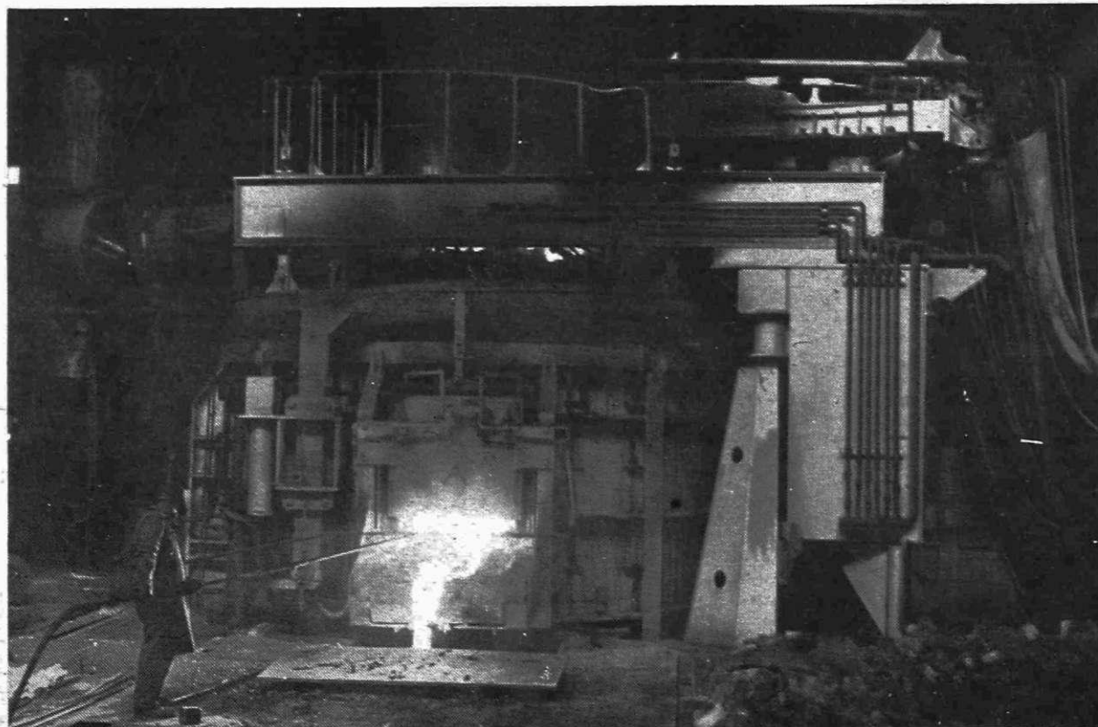
Sodelavec pri vpihovanju kisika v električno peč
