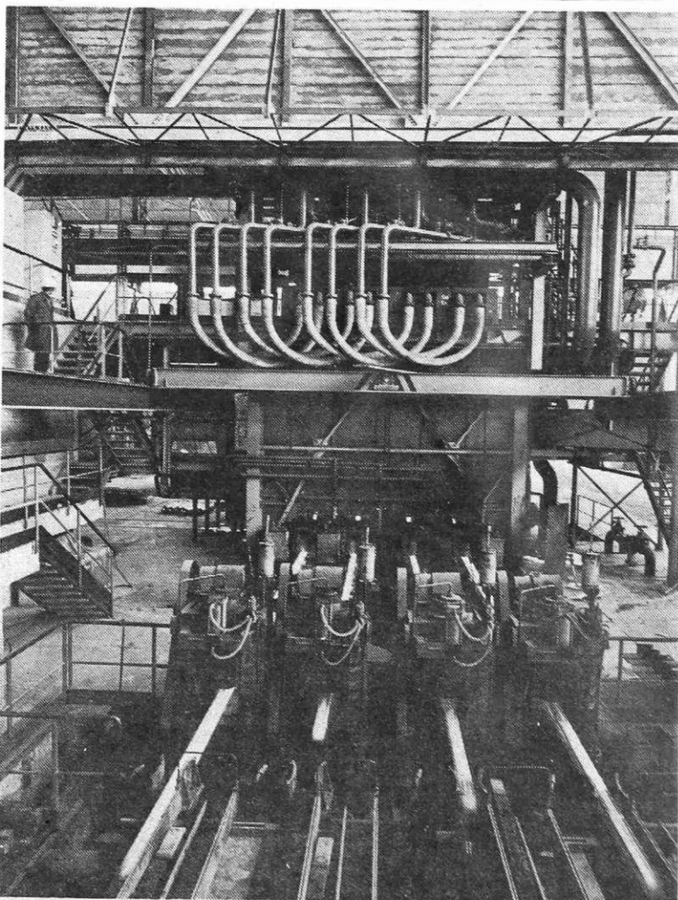
Električna peč v železarni Štore – konti naprava
