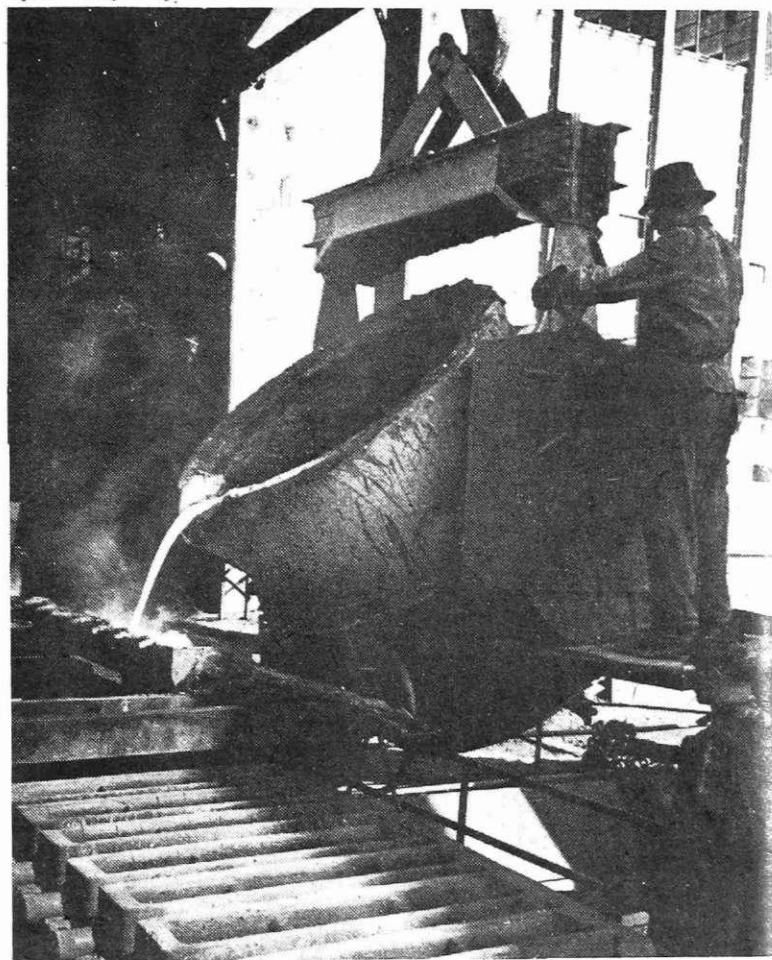
Izlivanje groblja na elektro plavžu v železarni Štore
