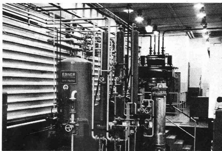
Vodikarna HVŽ - notranost strojnice.
