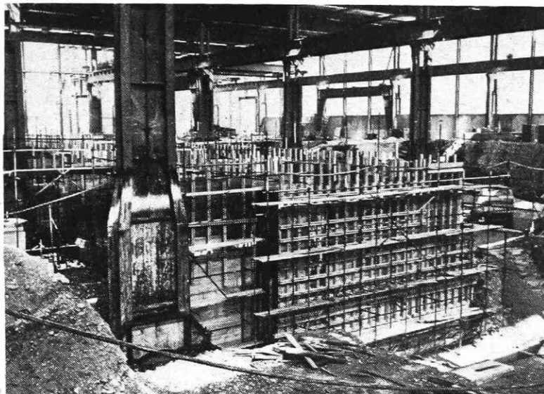
Dela na temeljih naprav nove hladne valjarne — 29. V.
