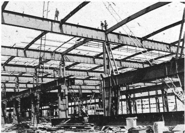
Stebrišča nove hladne valjarne na Belu - 29. V.
