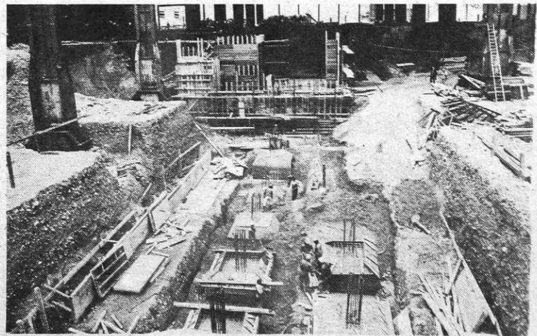
Betoniranje temeljev za naprave v novi hladni valjarni — 15. aprila
