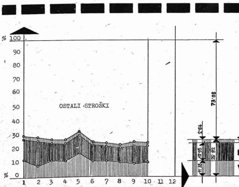
Diagram deleža stroškov vzdrževanja, energije in transporta v lastni ceni za tono blagovne proizvodnje za 10 mesecev
