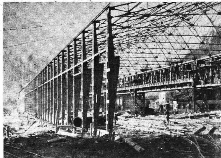
Montaža hale valjarne 2400 na Javorniku
