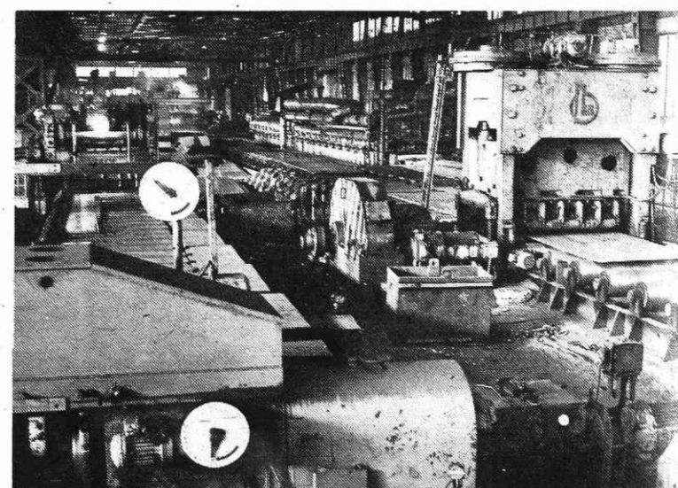
Del valjarne pločevine 2400 danes
