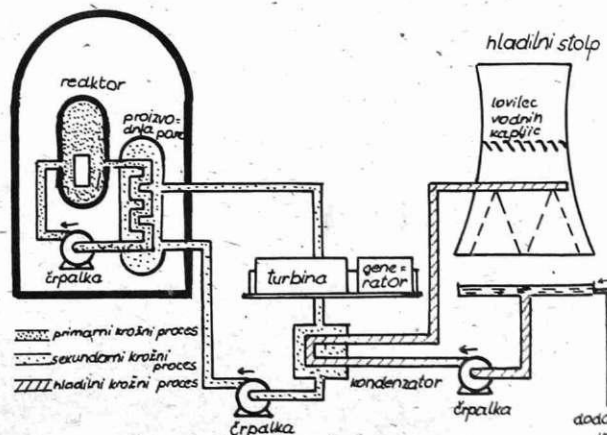
Shema hlajenja jedrske elektrarne z mokrim vodnim stolpom
