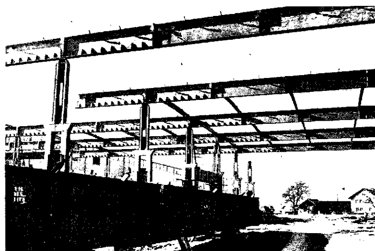
Vezi konstrukcije nove hladne valjarne — 11. 11.
