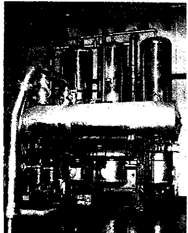
Centralna toplotna izmenjevalna postaja — toplotni izmenjevalci in ekspanzijske posode
