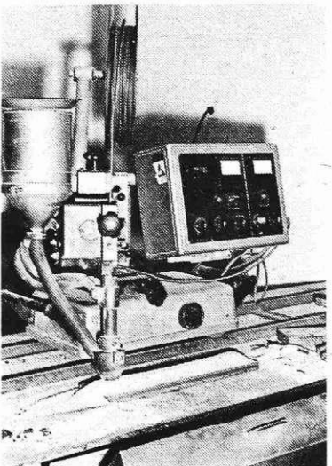
Aparat za varjenje pod praškom
