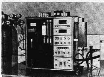
Aparat za določanje kisika in dušika v jeklu
