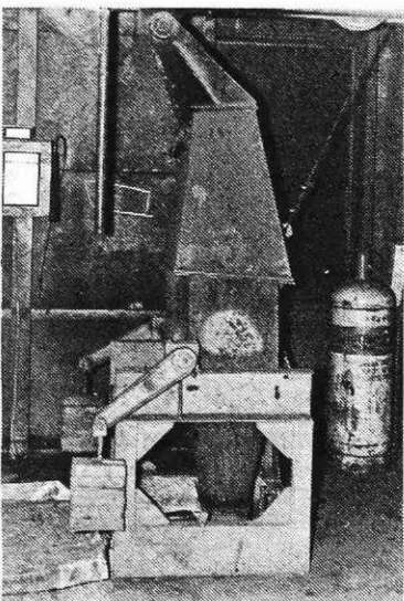
Eksperimentalna ponvica za sintranje
