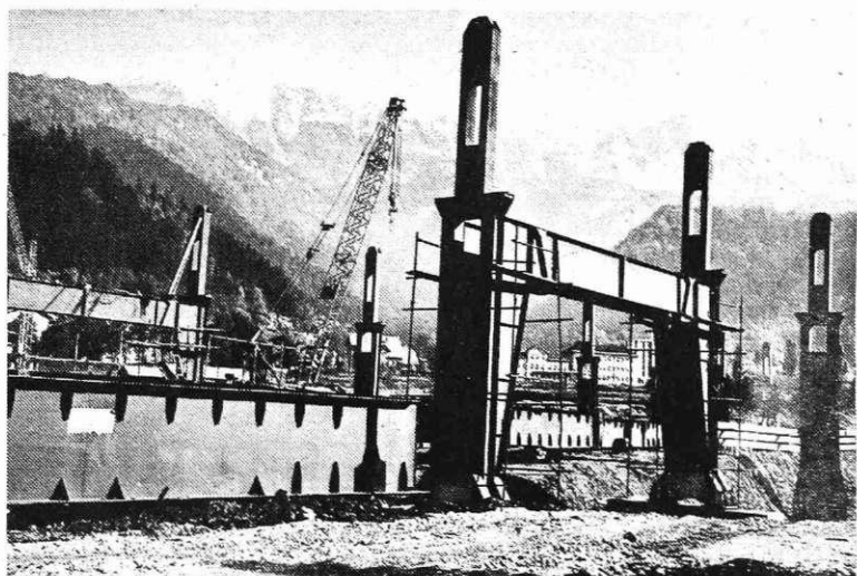
Zadnje dni na gradbišču nove hladne valjarne
