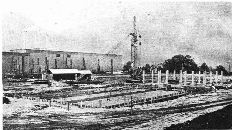
Polaganje armature in betoniranje za higienske prostore nove hladne valjarne na Beli
