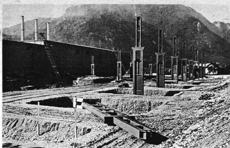
Zadnje dni na gradbišču nove hladne valjarne
