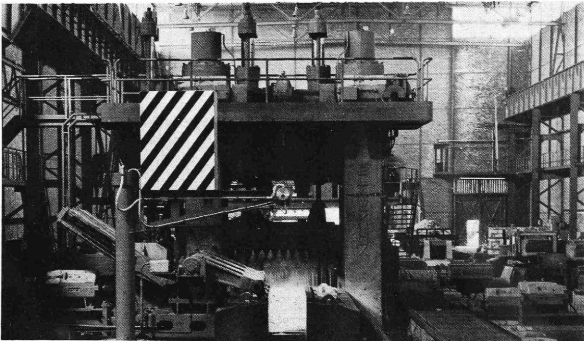
Valjanje na Blumingu
