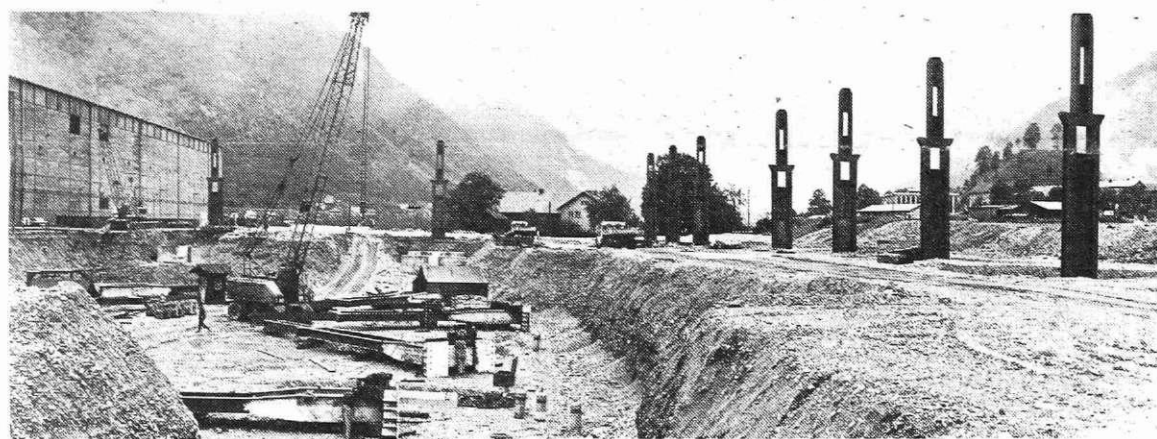
Zadnje dni na gradbišču nove hladne valjarne
