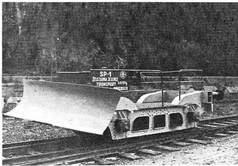
Autor tehničnega predloga Ivan Justin, je uspešno rešil izdelavo snežnega pluga za pluzenje širokotirnih naprav v Železarni (o tem smo poročali v zadnji številki Železarja)
