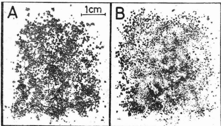
Slika 2: Primerjava zrnatosti našega in Lincolnovega varilnega praška
