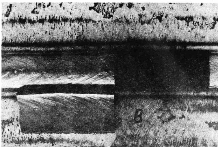
Slika 4: Izgled vara in varilne žilindre (Lincolnov prašek »780«)
