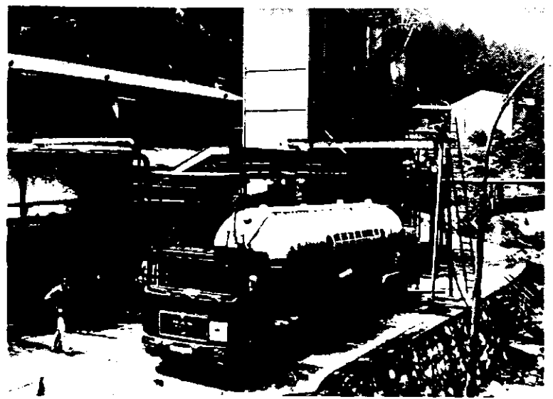
Autocisterna s katero smo v železarno dobili iz Zahodne Nemčije tekoči argon, ki smo ga uvozili za potrebe našega trga, ker domača proizvodnja ne pokriva povpraševanja. Kot zanimivost naj navedemo, da je bruto teža cisterne 36 ton v kateri se prevaža 14 ton tekočega argona pod temperaturo minus 186 stopinj Celzija
