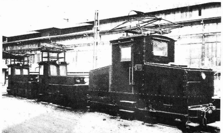
Na sliki so ozkotirne električne lokomotive, ki so zadnje obratovali v javorniških obratih. Obe električni lokomotivi OE-IV in OE-V sta bili kupljeni 1948. leta, desna akumulatorska OE-VI pa je bila leta 1950 izdelana v naši železarni po vzorcu ELIN-ove lokomotive (OE-II, 1932), ki sedaj prevaža tekoči grodelj od plavžev k martinovim pečem.
