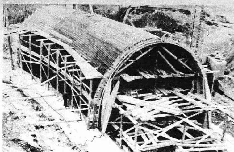
Čez potok Bela je narejen opaž za betonski most preko katerega bo tekla nova cesta, ki jo sedaj urejajo od Potok do Javornika.
