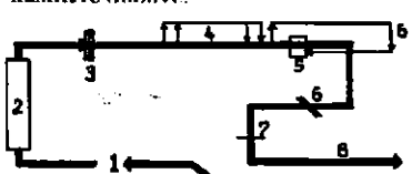
Slika 1: 1 — priprava vložnega materiala, 2 — ogrevanje, 3 — valjanje, 4 — termična obdelava, 5 — valjanje, 6 — rezanje, 7 — pregled — tehtanje, 8 — odpravljanje.
