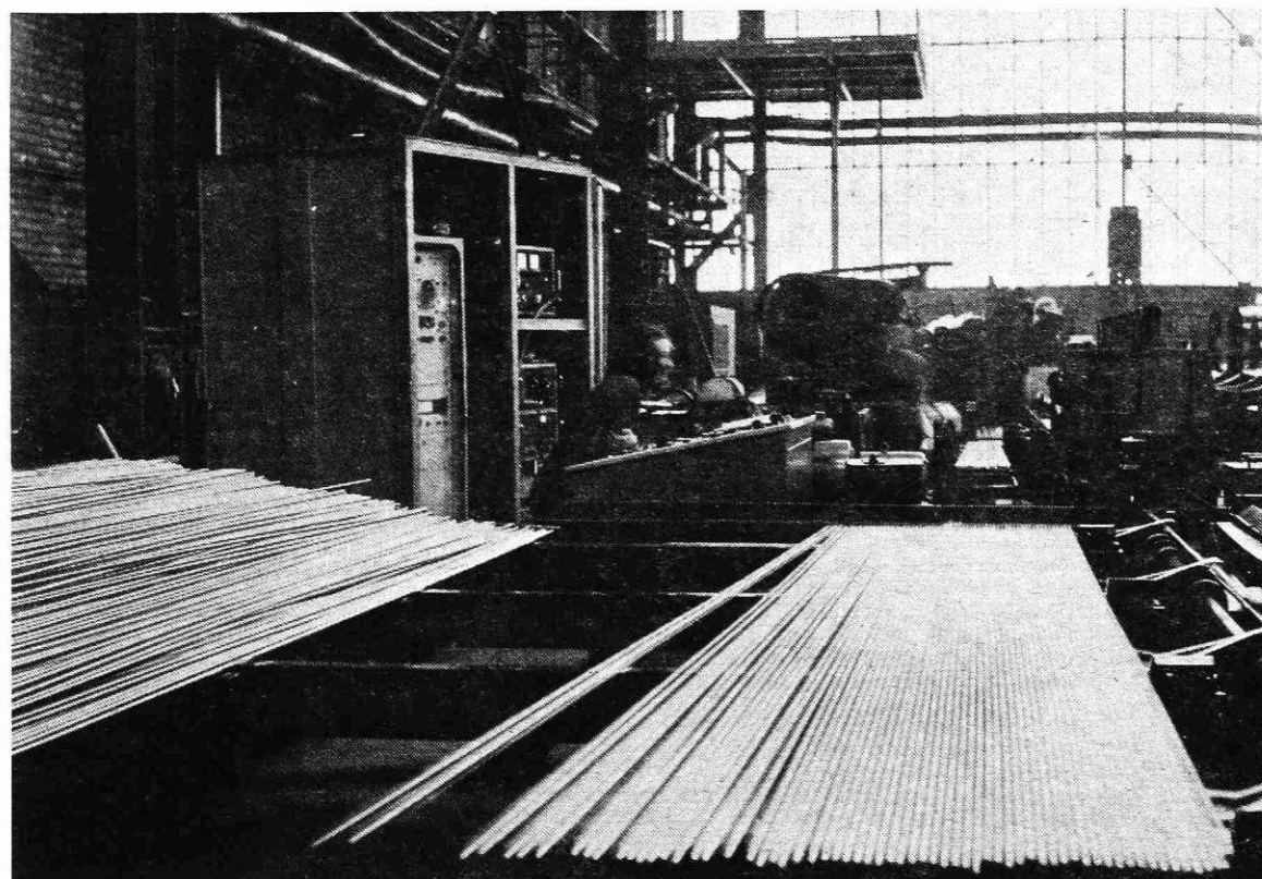
Sodelavka pri avtomatski kontroli jekla v jeklovleku
