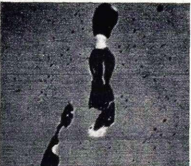
Slika 5 — Oblika in porazdelitev vključkov svinca v avtomatskem jeklu (elektr. slika pov. 420)
