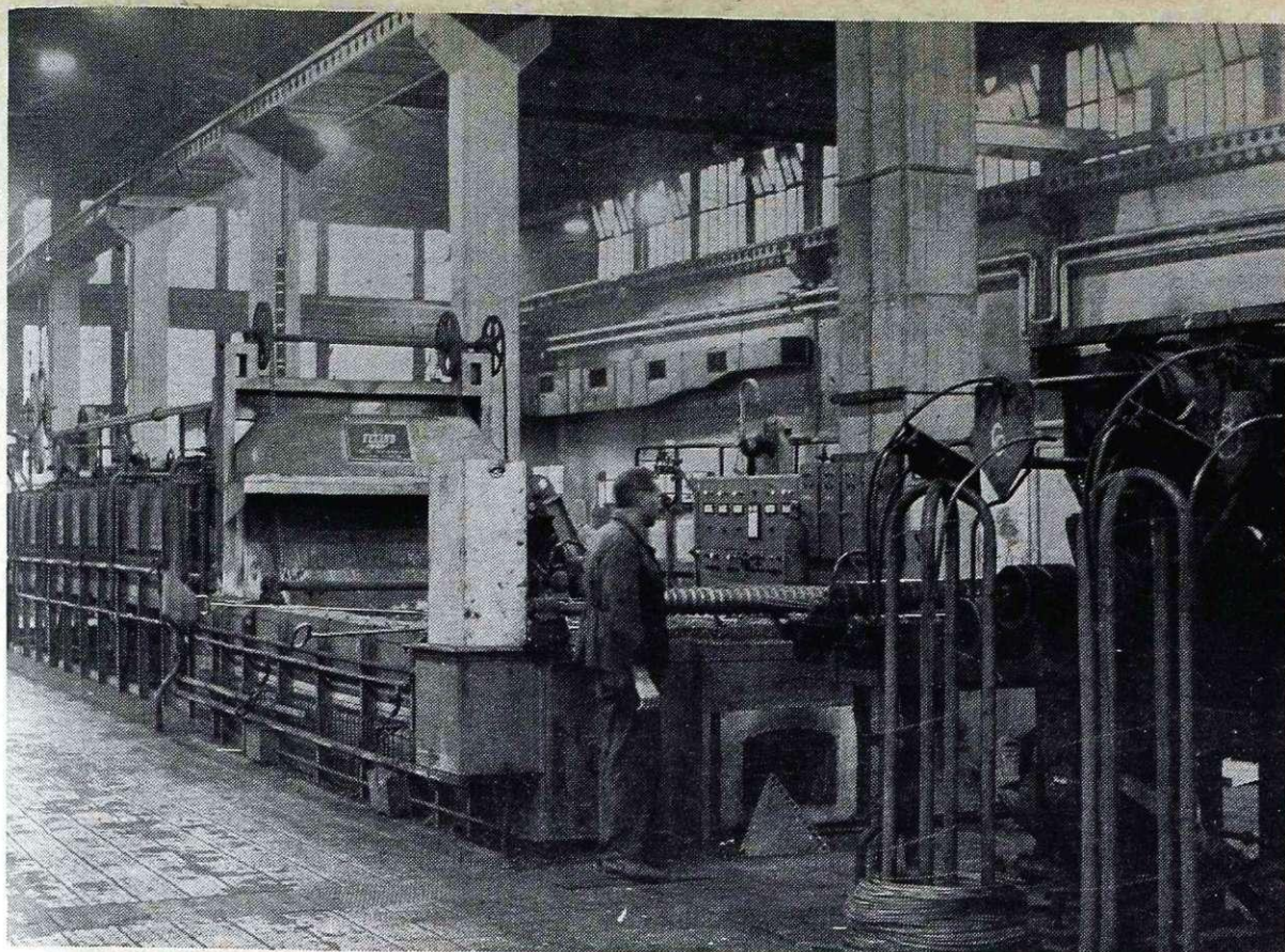
ŽIČARNA — naprave za patentiranje žice
