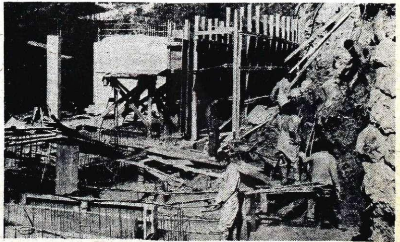
Delavci SGP Save grade-tih poleg doma dr. Franceta Berglja na Zgornjem Plavžu apartmanjsko, garsonjersko zgradbo, kjer bodo prebivali ostareli občani, samski in zakonci, ki so še sposobni sami skrbeti zase. Lahko pa bodo hrano in drugo pomoč dobivali tudi v domu. Graditve objekta na tem ozkem prostoru je precej zahtevna, ker so morali prestaviti električni vod, poleg tega bodo morali s tem teren pad ceste v Planino pad Golica zavarovati z opornim zidom. Predvidevajo, da bo zgradba nared prihodnje jesen, večjala pa bo blizu pet milijonov dinarjev.
