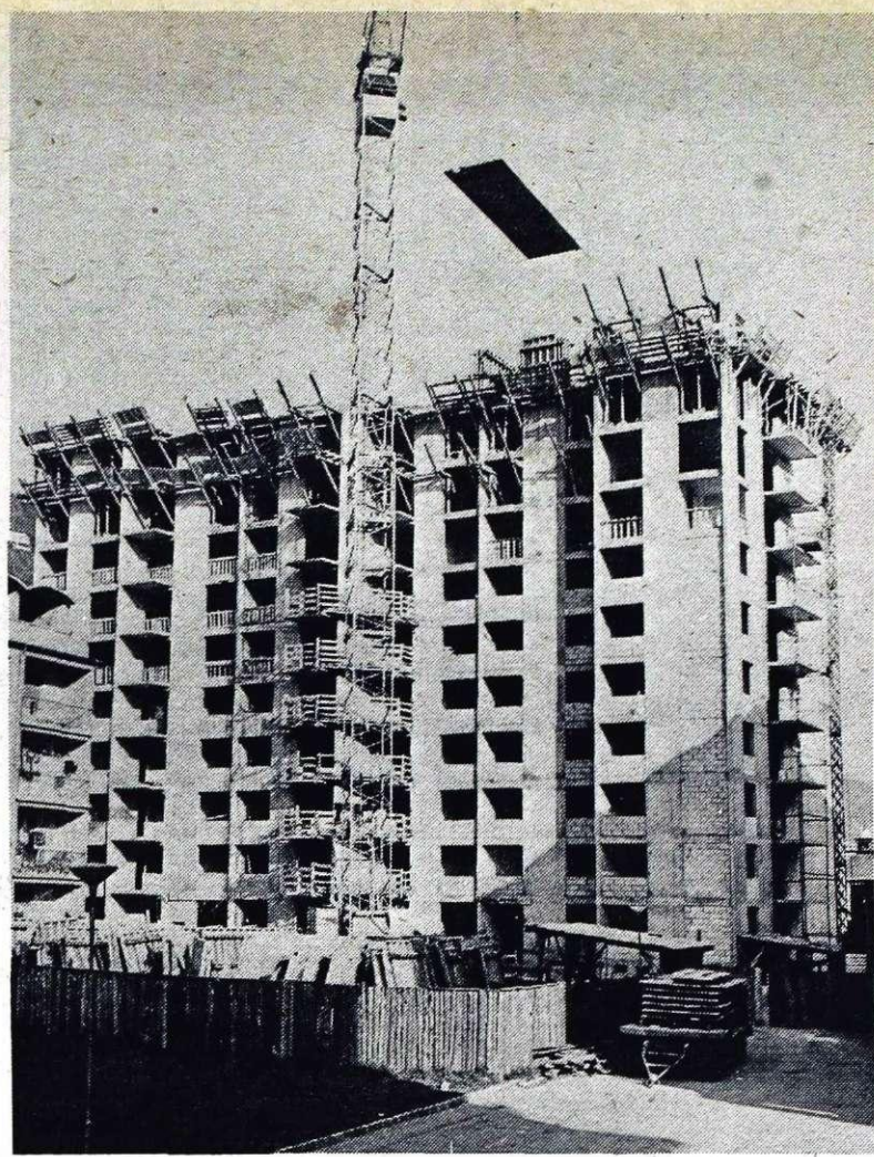
Pred našimi očmi z veliko naglico raste največji stanovanjski objekt na Jesenicah. Delavci SGP Save z uporabo novega polmontažnega sistema Omnia dokončujejo zadnji dve etaži dvanajst nadstropne členjene stolpnice.
