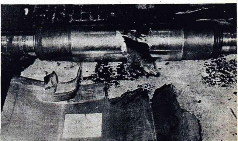
Pogosti primeri nekvalitetnih vroč valjanih trakov iz kaljarne Bela, povzročajo velike težave pri hladni predelavi in škodo zaradi okvar delovnih valjev Sicmag valjenega stroja.
