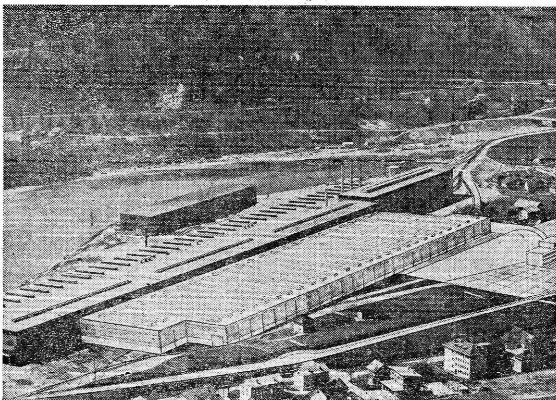
Valjarna Bela z vrisano shemo bodoče hladne valjarne
