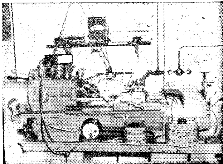
Raziskovalni oddelok — naprava za določevanje sposobnosti deformacije jekla v vročem
