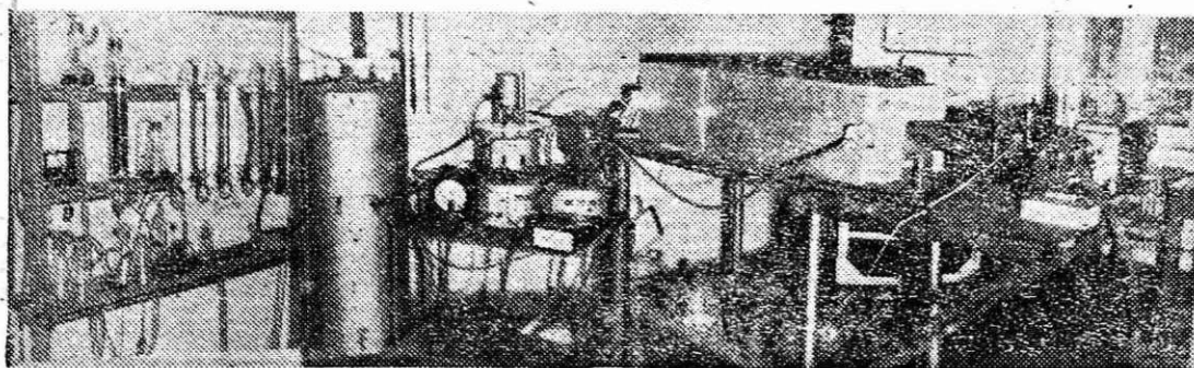
Laboratorij za žarenje v zaščitni atmosferi
