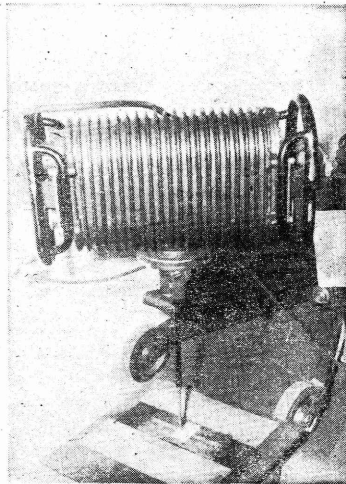
Rentgen — določevanje homogenosti zvara
