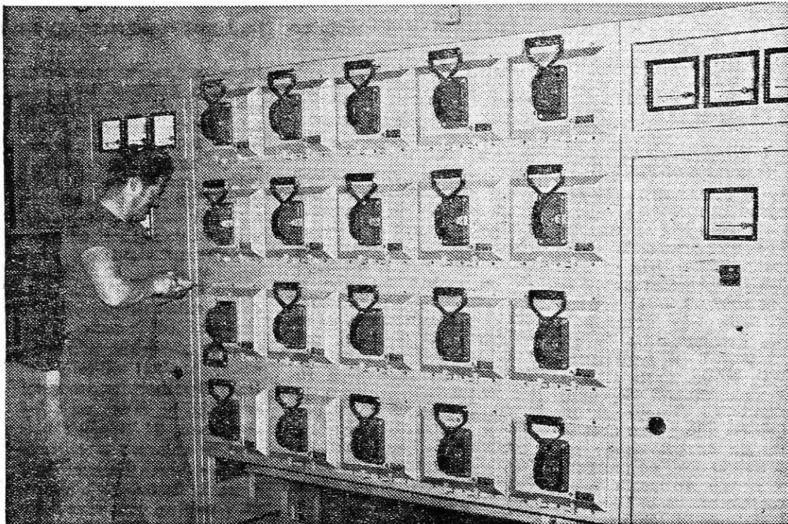
Stikalno razdelilna omara, proizvod ELIMA za našo železarno
