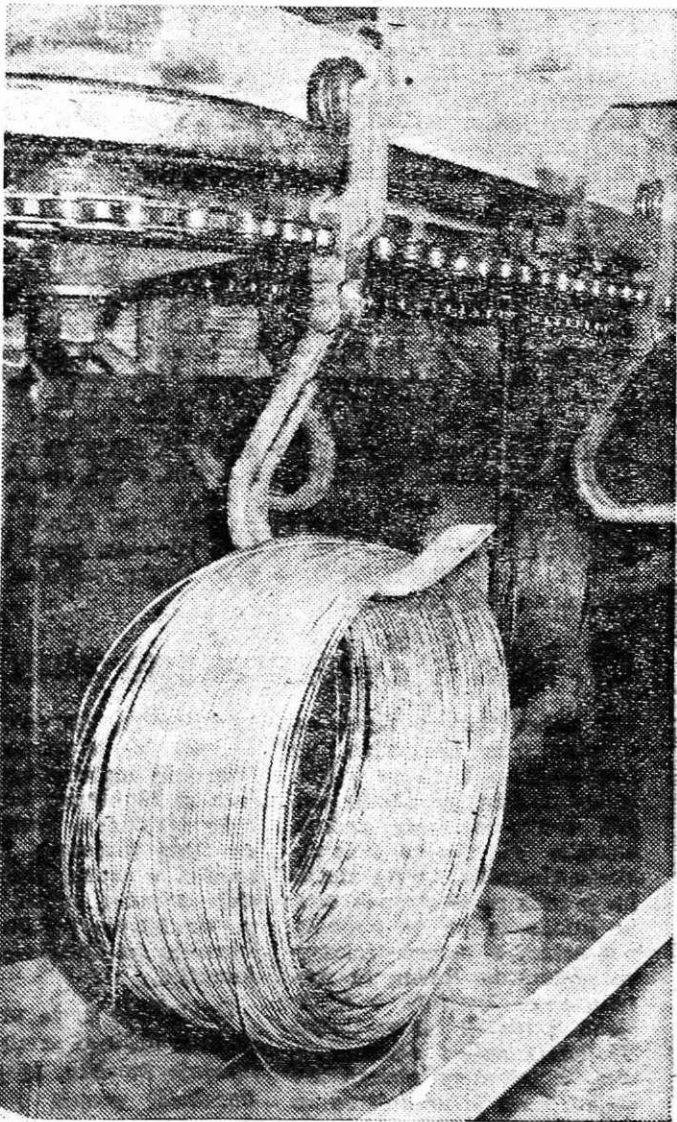
Valjarna žice — žica na tekočem traku
