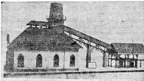
Maketa javorniškega plavža, ki jo hrani tehnični muzej na Dunaju
