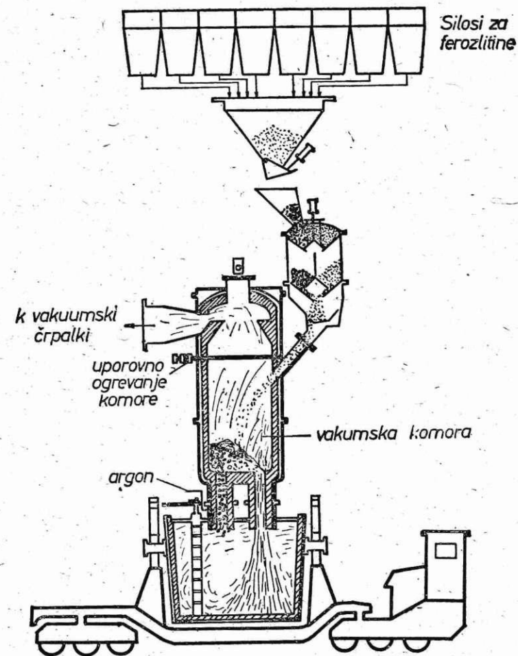
RH — vakuumska naprava
