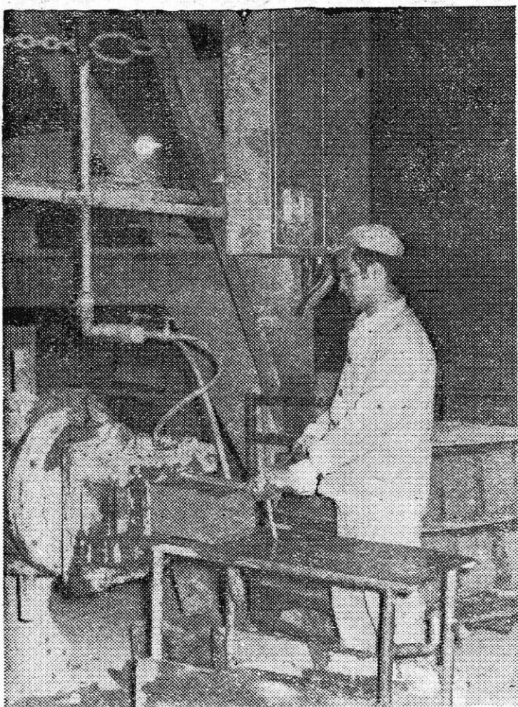
Sodelavec pri oblikovanju ognjestalne opeke v šamotarni
