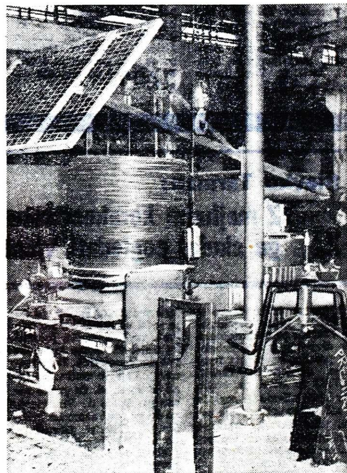
V žičarni so te dni začeli poskusno obratovati na novem žičarskem stroju TM 3 firme Redaelli za hladno vlečenje žice.
