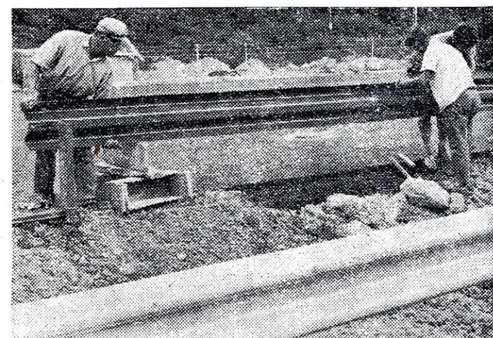
Delavci pri montaži cestnih odbojnikov izdelanih v naši železarni na avtocesti Vrhnika—Postojna
